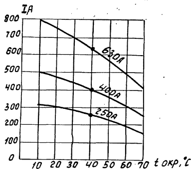
Рис. 7.2. Кривые зависимости допустимой нагрузки на шинопровод ШРА73 на 250, 400 и 630 А от температуры окружающей среды.
