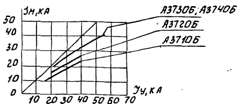
Рис. 5-1. Напряжение 380В
