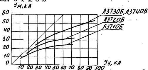
Рис. 5-1. Напряжение 380В
