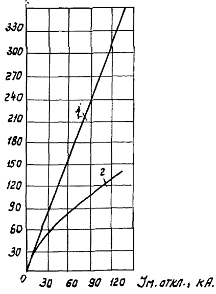
Рис. 1.2. Напряжение 380В, \cos\varphi = 0,2 , 1600А
