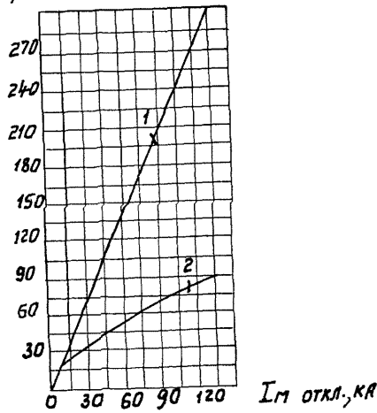
Рис. 1.4. Напряжение 380В, \cos \varphi = 0,2 , 1000А
