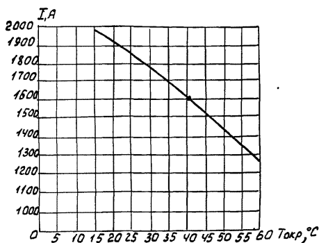
Рис. 7.1. Кривая зависимости допустимой нагрузки на шинопровод ШМА73 на 1600А от температуры окружающей среды.
