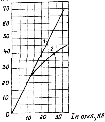
Рис. 1.3. Напряжение 660В, \cos \varphi = 0,3 , ток 1000А
