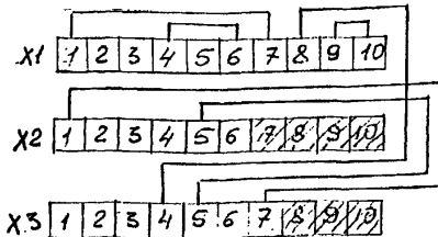
Рис.1 Электрическая принципиальная схема управления переверткой электроприводом насоса маслобака для режимов "опробование" и "Работа".
