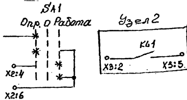
Рис.1 Электрическая принципиальная схема управления переверткой электроприводом насоса маслобака для режимов "опробование" и "Работа".
