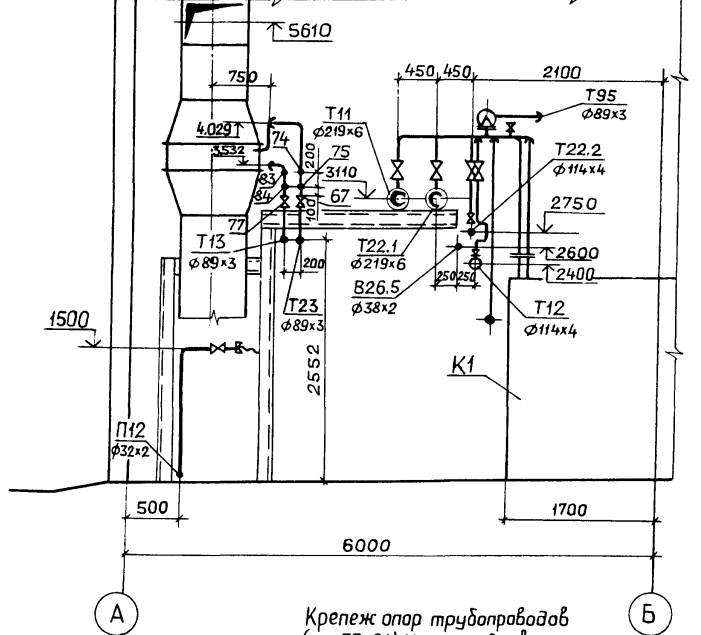
РАЗРЕЗ 5-5, ЛИСТ ТМ-18
