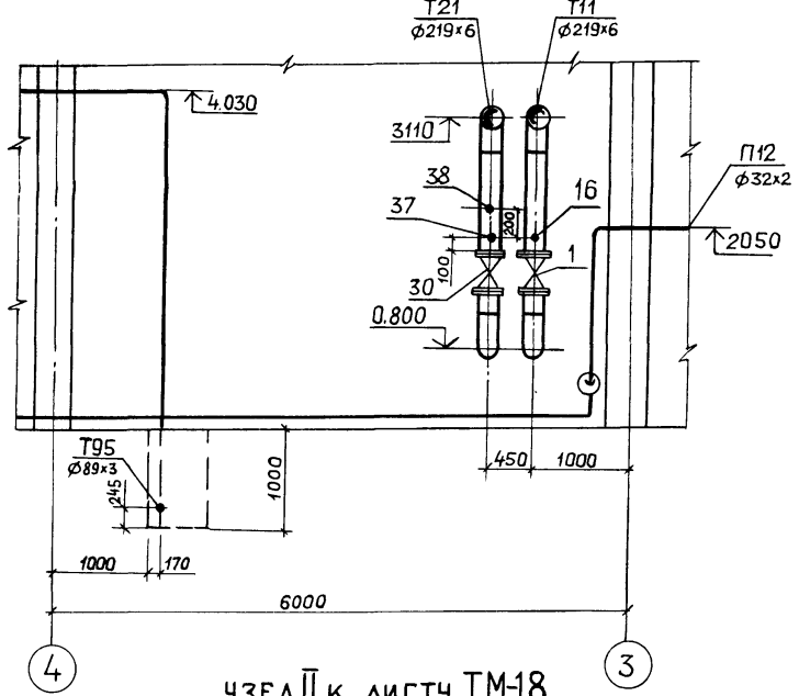
УЗЕЛ II к листу ТМ-18
