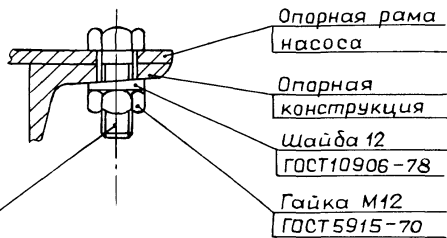
КРЕПЛЕНИЕ I
