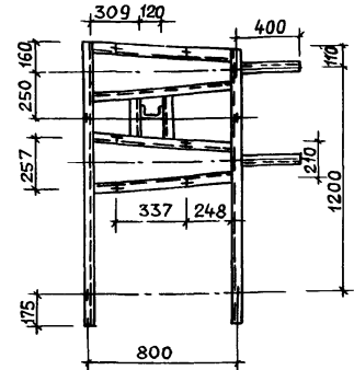
ПЛАН ОПОРНОЙ КОНСТРУКЦИИ
