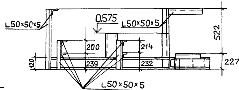
ПЛАН ОПОРНОЙ КОНСТРУКЦИИ
