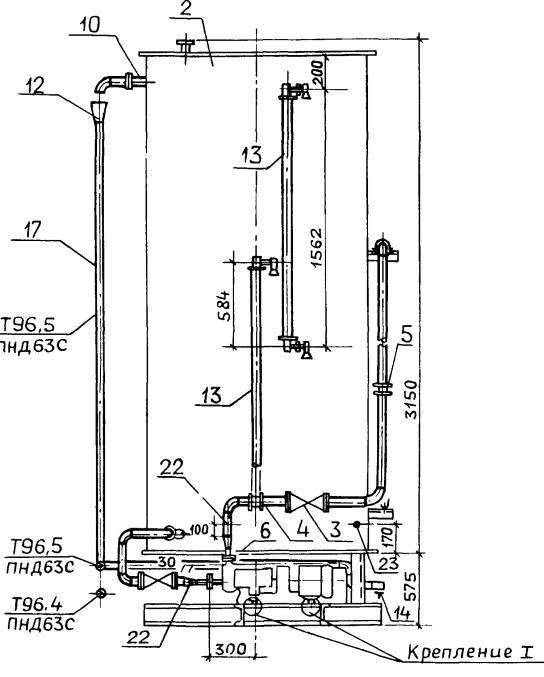
СХЕМА
