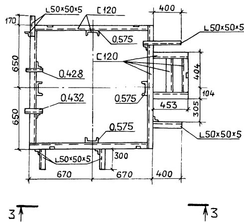
ПЛАН ОПОРНОЙ КОНСТРУКЦИИ
