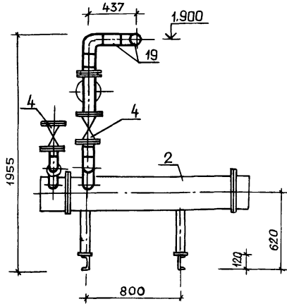
РАЗРЕЗ 3-3
