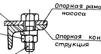
КРЕПЛЕНИЕ I
