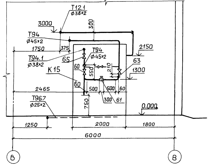
РАЗРЕЗ 2-2, ЛИСТ ТМ-18
