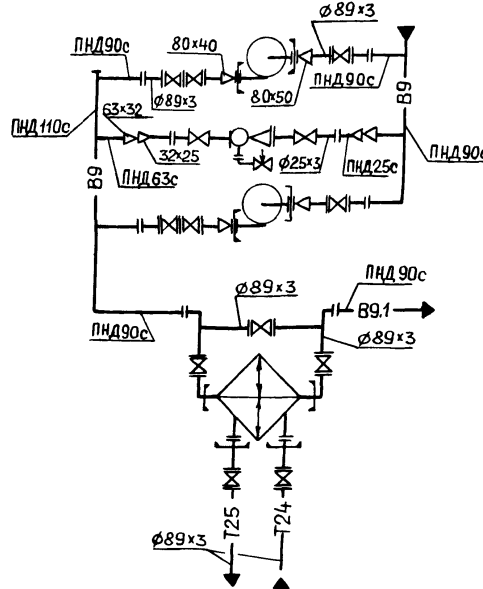
СХЕМА
