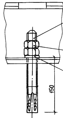
КРЕПЛЕНИЕ II
