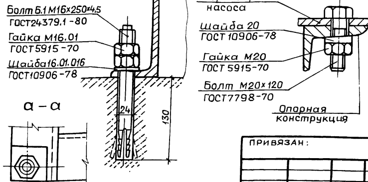
КРЕПЛЕНИЕ I
