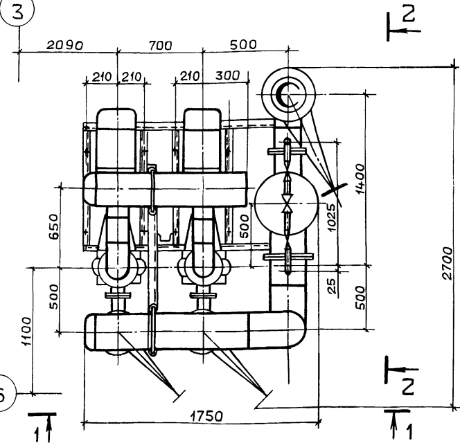
ПЛАН
