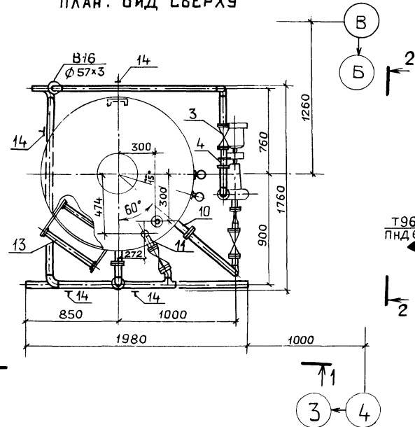
ПЛАН. ВИД СВЕРХУ
