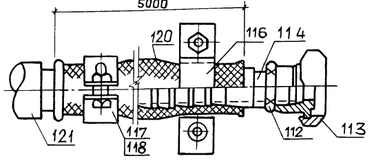
УЗЕЛ II к листу ТМ-18
