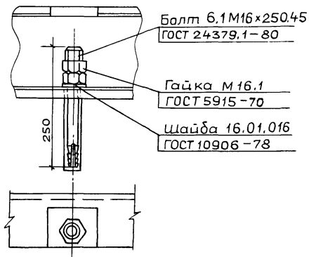
КРЕПЛЕНИЕ II
