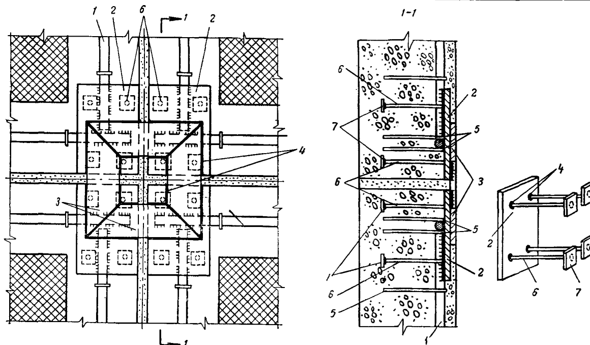
Рис. 5. Пример решения детали стыкования арматуры ребристых панелей
