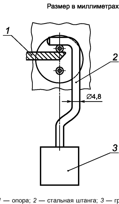
Рисунок 14 — Установка для испытания трубчатых штырей
