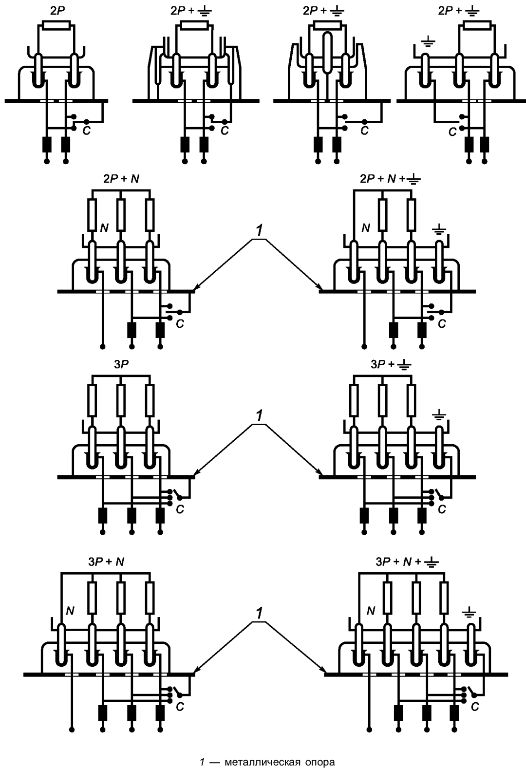
Рисунок 17 — Схема соединения для испытания на нормальную работу
