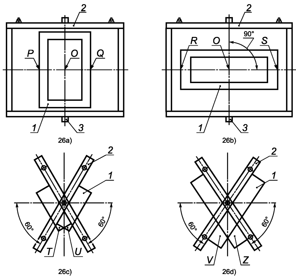
1 — образец; 2 — лист фанеры; 3 — ось поворота
