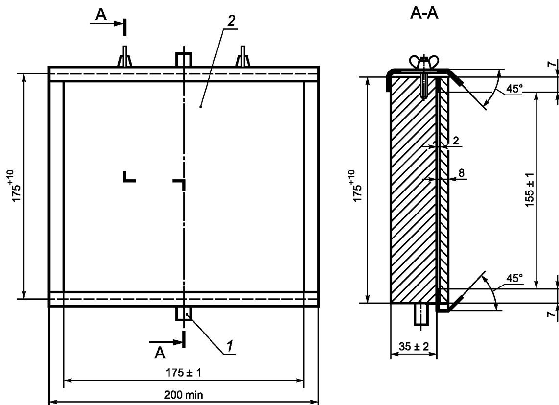
Рисунок 24 — Монтажная опора
