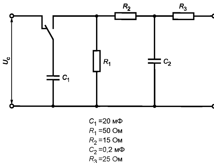
Рисунок В.1 — Схема испытательного генератора импульсов
