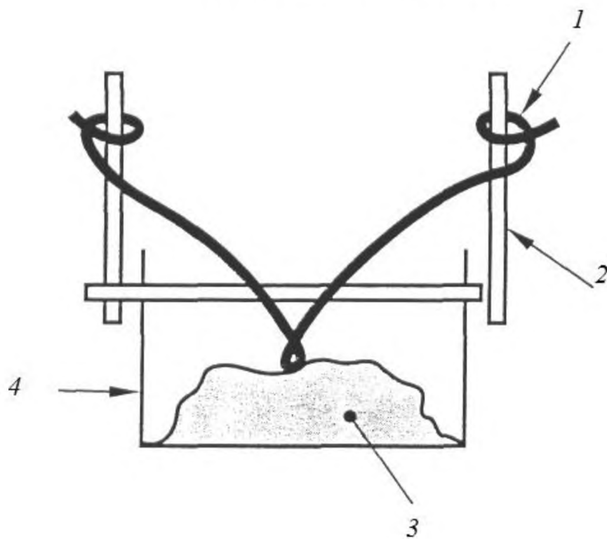
1 1 – проволока для поджига; 2 – электроды; 3 – образец; 4 – тигель
