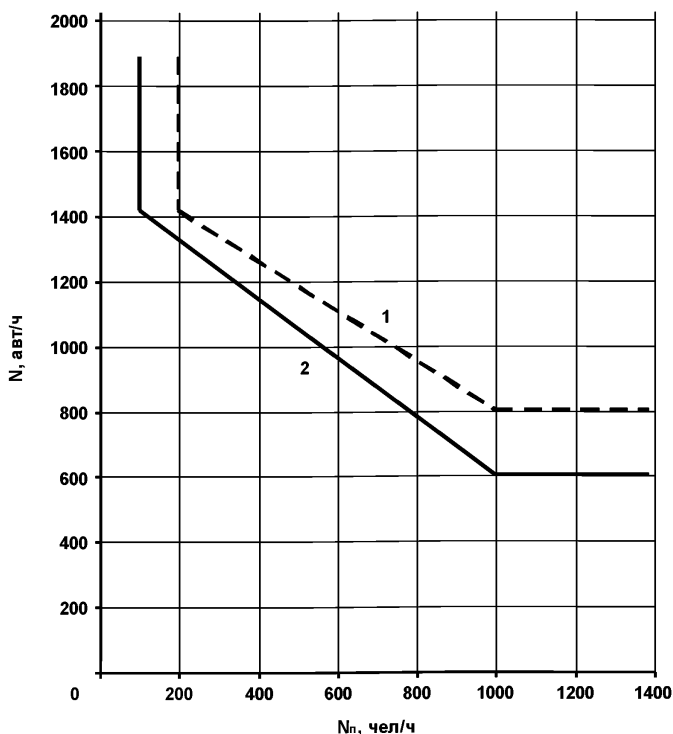
Рисунок 19 - График для определения необходимости установки пешеходных светофоров вызывного действия на пешеходных переходах 1 – с островком безопасности; 2 – без островка безопасности; N – интенсивность движения транспортных средств; N_p – интенсивность пешеходного движения
