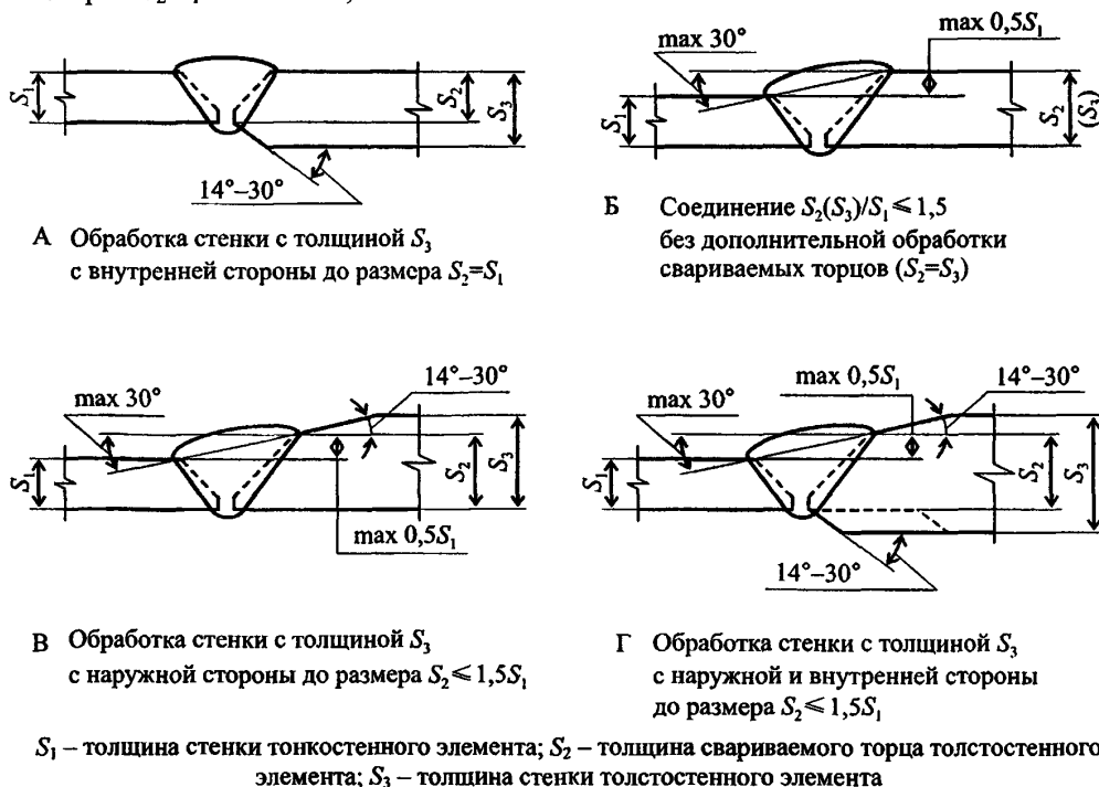
Рисунок 9.2 – Регламентируемые варианты обработки торцов стыкуемых разнотолщинных элементов
