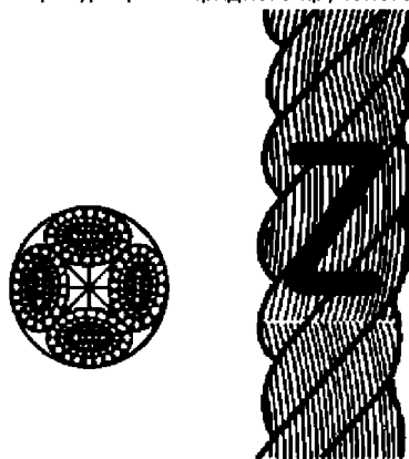
Рисунок 1 — Конфигурация 3-рядного крученного каната (тип А)
