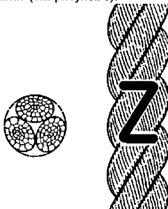
Рисунок 1 — Конфигурация 3-рядного крученного каната (тип А)
