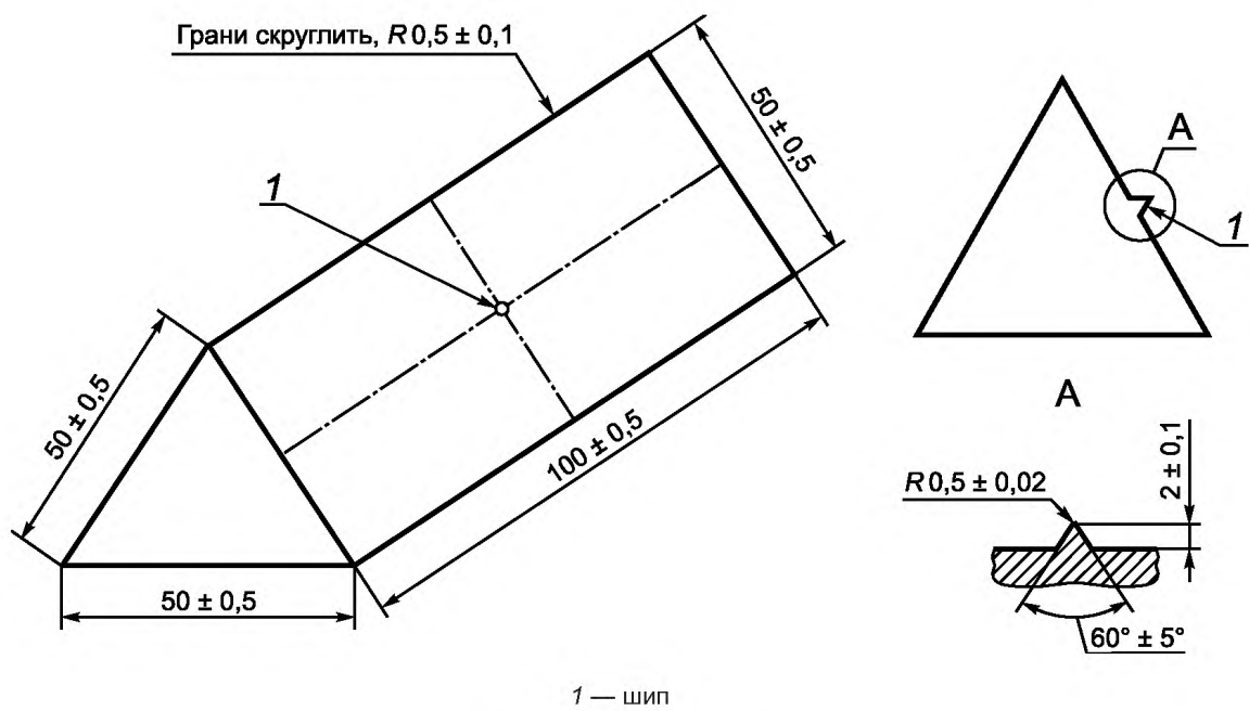
Рисунок 14 — Оправка
