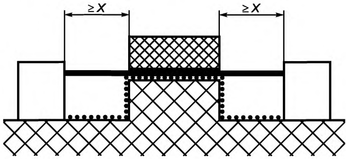
Рисунок Е.5 — Несплошной стык с узкими канавками
