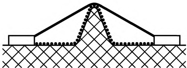
Рисунок Е.3 — V-образная канавка
