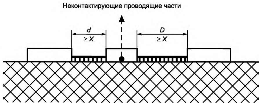
Расстояние изоляции с интервалом; проводящая часть, не имеющая соединения. Зазор — это расстояние (d + D) , путь утечки — также (d + D) . Если величина (d + D) менее чем X , ее значение принимают равным нулю.
