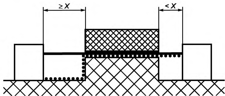
Рассматриваемый путь включает в себя несплошной стык с канавкой с одной стороны, имеющей ширину менее X мм, и с канавкой с другой стороны, имеющей ширину 1 мм и более. Зазор и расстояние утечки определяют, как показано на рисунке Е.7.
