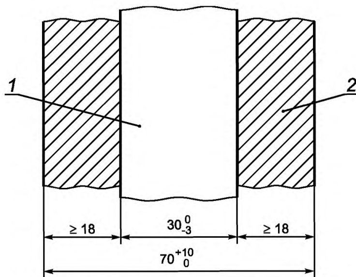
Рисунок 16 — Конечное положение оправки
