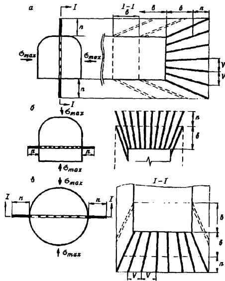
Рисунок 11— Схемы камуфлетного взрывания по рядам шпуров:
