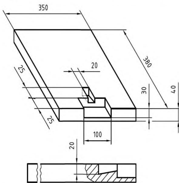
Рисунок 1 – Пластина с пазом для измерения времени гелеобразования
