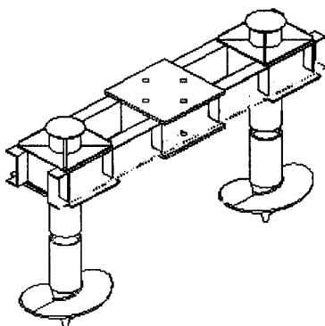
Рис. 4.3 - Стальной сварной ростверк фундамента типа 2Ф500-219-6-24-4 из стали класса С345: балка из двух швеллеров №24 с опорной плитой и 4-мя отверстиями диаметром 42 мм с двумя нижними и двумя верхними опорными столиками
