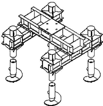
Рис. 4.5 - Стальной сварной ростверк фундамента типа 4Ф500-219-6-24-4 из стали класса С345: балка из двух швеллеров №24 с опорной плитой и 4-мя отверстиями диаметром 42 мм, опёртая на две нижних балки с опорными столиками
