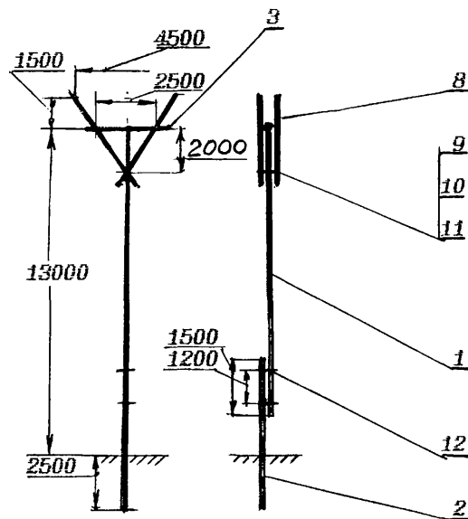
Защита одностоечная
