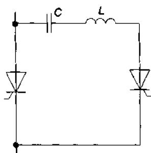
Рисунок А.1b — Пример контура коммутации
