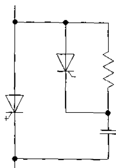
Рисунок А.1d — Пример гасящего контура Рисунок А.1 — Примеры форм сигнала и их контуров
