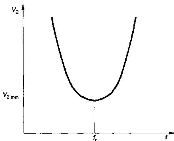
Рисунок С.2 — Взаимосвязь между напряжением на конденсаторе и подаваемой частотой
