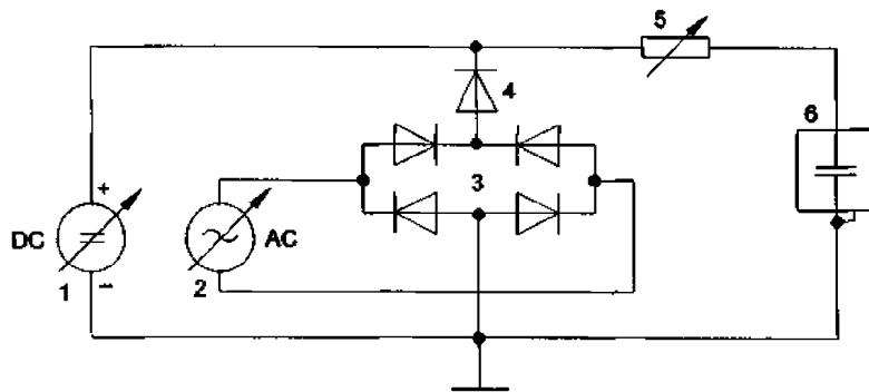
Рисунок 2 — Источник постоянного тока N — Тип 1
