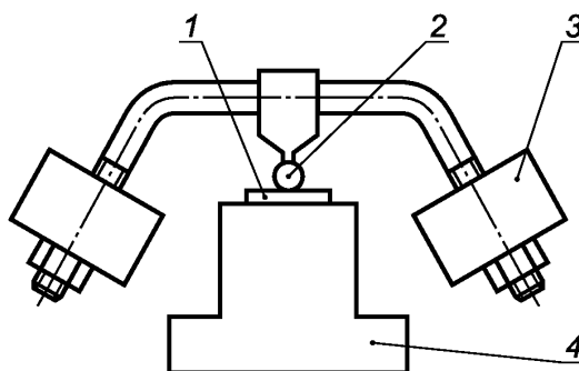
1 — испытываемый образец; 2 — шарик давления; 3 — груз; 4 — опора для образца
