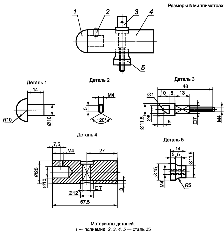
Рисунок 19 — Ударный элемент маятникового молотка для нанесения удара
