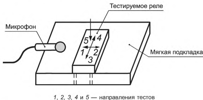
Рисунок 14 — Установка для теста излучения акустических шумов
