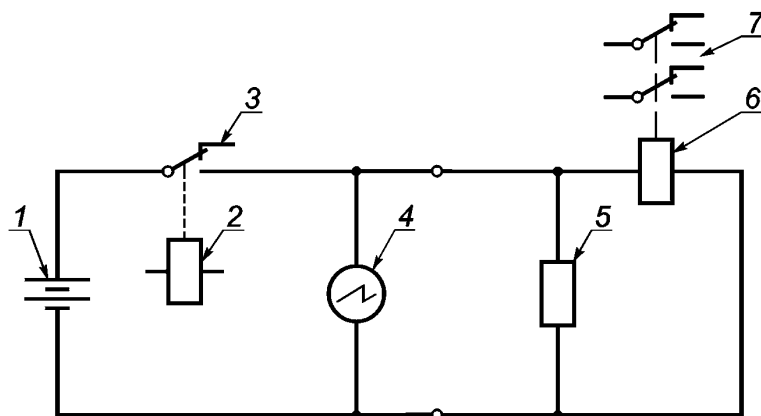
1 — подача возбуждения (низкий импеданс); 2 — катушка индуктивности коммутационного реле; 3 — контакт коммутационного реле (без дребезга); 4 — мониторный прибор (осциллограф); 5 — схема подавления помех; 6 — катушка индуктивности испытуемого реле; 7 — контакты испытуемого реле
