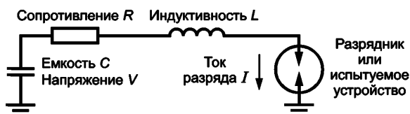
Рисунок 5 — Принципиальная схема устройства для моделирования разрядов статического электричества
