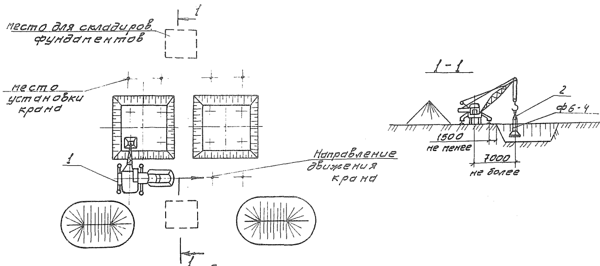
Рис. 2-2. Схема установки ж.б. фундаментов в грунтах II группы 1. Кран автомобильный КС-4561А 2. Строп 2СК-8,0/РТИ-8,0/КИ-6,3/2500 ОСТ 24.09048-79
