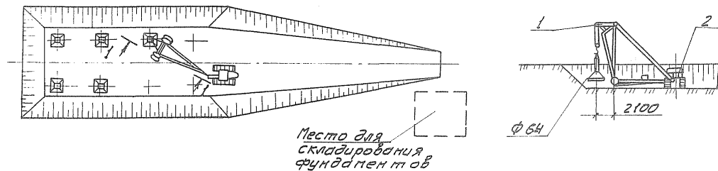
Рис. 2-1. Схема установки ж.б. фундаментов в грунтах I группы
