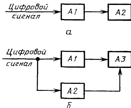
Рис. 1. Схемы проверки основной погрешности поверяемого прибора: А1—поверяемый прибор; А2—образцовое средство измерений напряжения (тока); А3—измеритель разности сигналов
