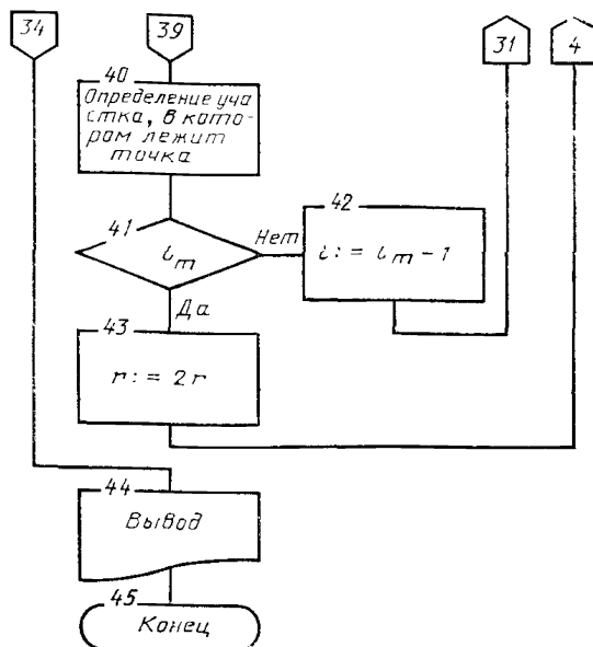
Рис. П. 23. Блок-схема программы проверки систематической составляющей погрешности поверяемого прибора, работающего в двоичном коде, и поиска проверяемых точек.
