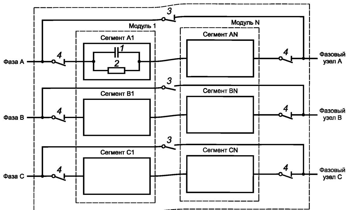
Рисунок 1 — Составные части батареи из последовательных конденсаторов
