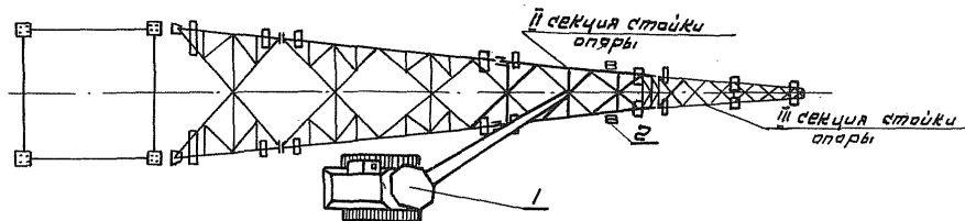
Рис. 14 Сборка II секции стоек опоры типа У2+5
