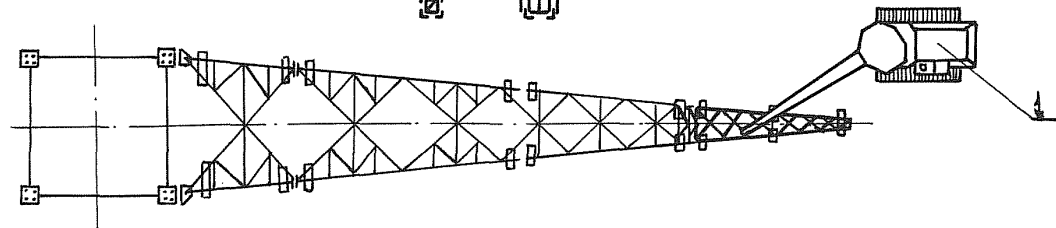
Рис. 13 Сборка III секции стойки опоры типа У2+5
