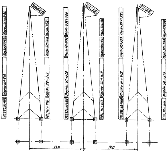
Рис.11 План расположения пакетов с деталями опоры У2+5 на пикете
