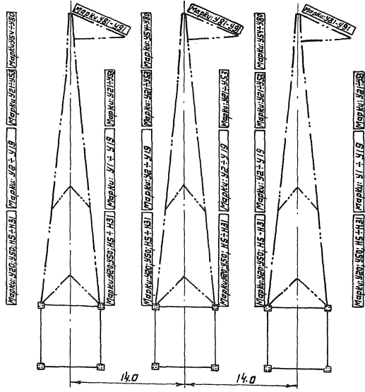
Рис. 20 План расположения пакетов стрелами опоры У2+12 на пикете
