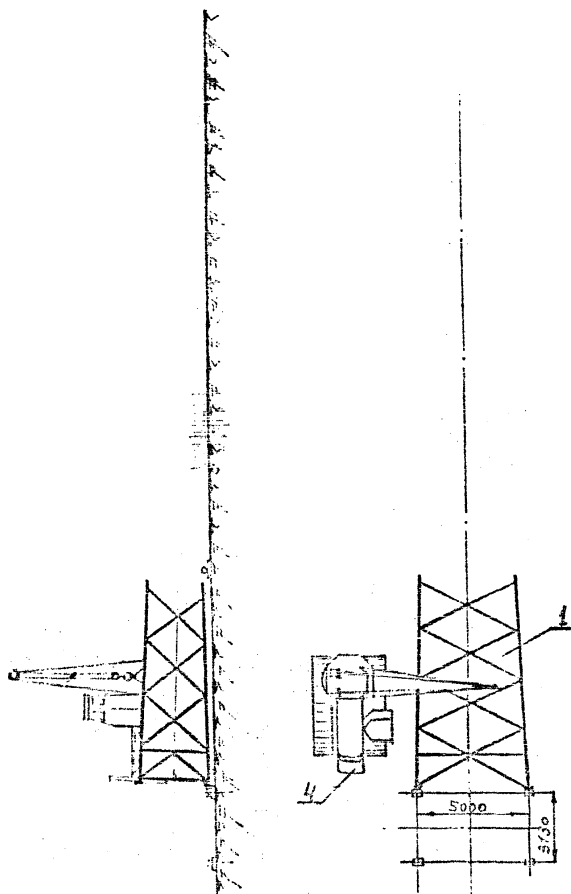
Рис. II Сборка 100 секции стбала опоры П220-3
