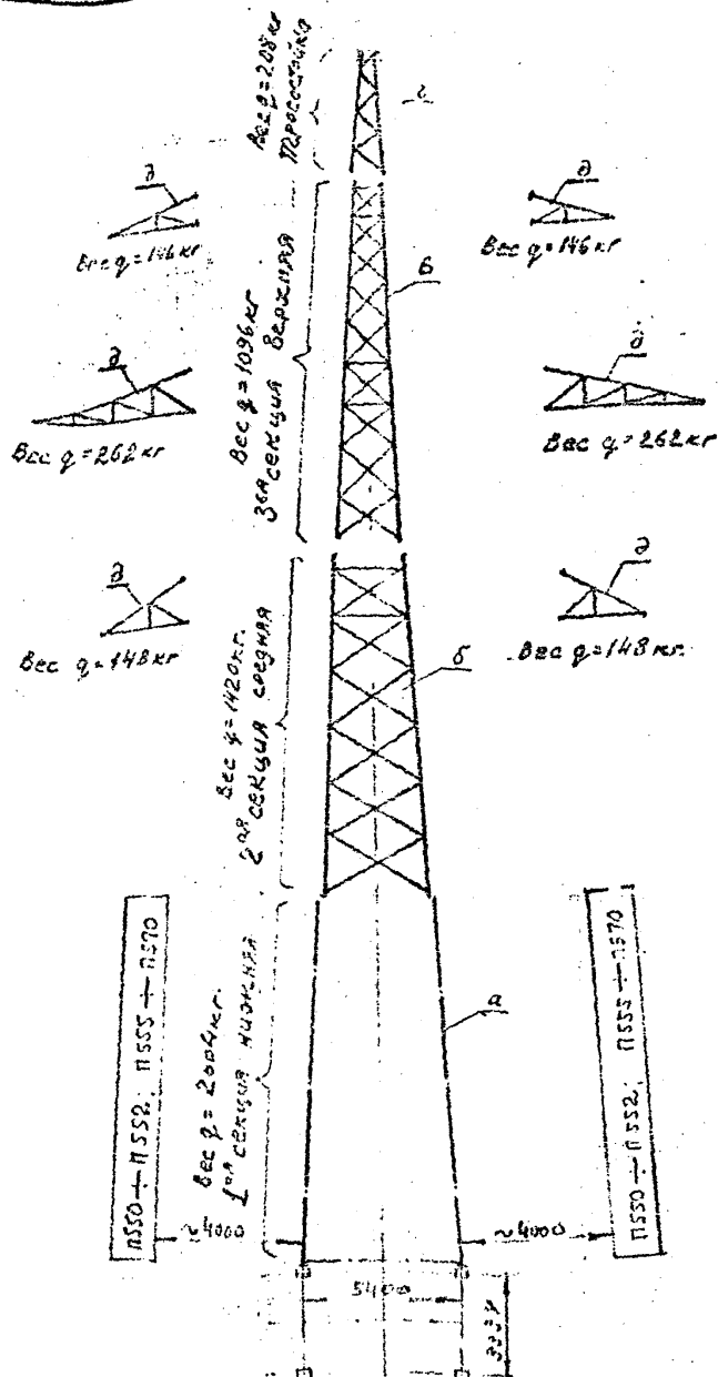
Рис. 23 Раскладка пакетов и секций опоры П220-2 на пикетисе а) 1 я секция нижняя; б) 2 я секция средняя; в) 3 я секция верхняя, г) Платформы.
