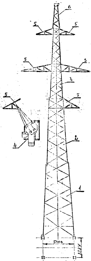
Рис. 27 Пристыковка траверсы и тросостойки к стволу опоры ПРЭО-2
