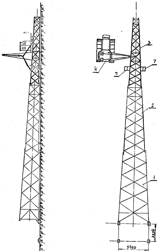
Рис. 26 Пристыковка 3 ей секции ствкола опоры П 220-2
