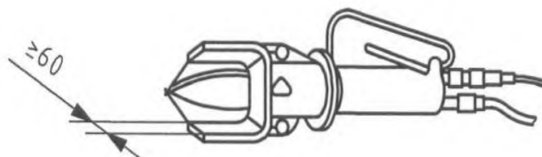
Рисунок 12 – Неподвижное защитное ограждение на ножницах/клещах для отрезания свинных ножек
