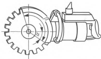
Рисунок 10 – Неподвижное защитное ограждение циркулярной пилы
