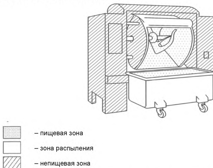
Рисунок 3 – Гигиенические зоны смесителя с горизонтальными валами
