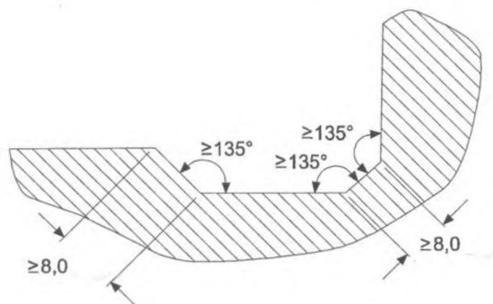
Рисунок В.3 – Углы в пищевой зоне
