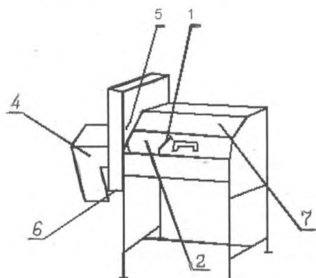
Рисунок 3 – Опасные зоны ломтерезки с разгрузочным коробом
