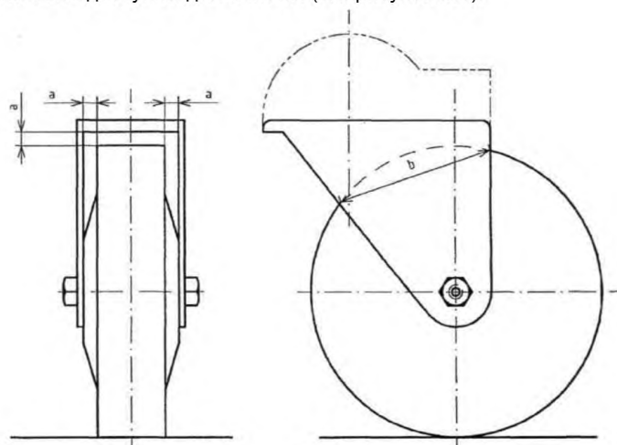
Рисунок В.6 – Примеры размеров
