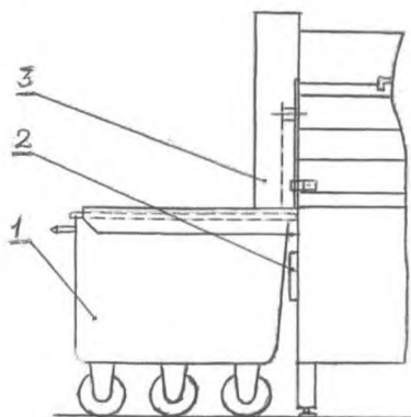
Рисунок 6 – Ломтерезка с разгрузочным лотком. Меры защиты
