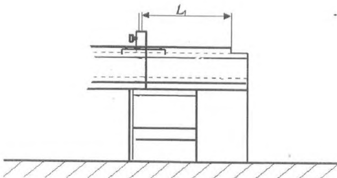
Рисунок 5 – Ломтерезка. Безопасные размеры
