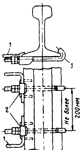
Рис. 3 Присоединение к тяговому рельсу проводников защитного заземления: 1 — провод заземления; 2 — зажим заземления; 3 — крепежной болт
