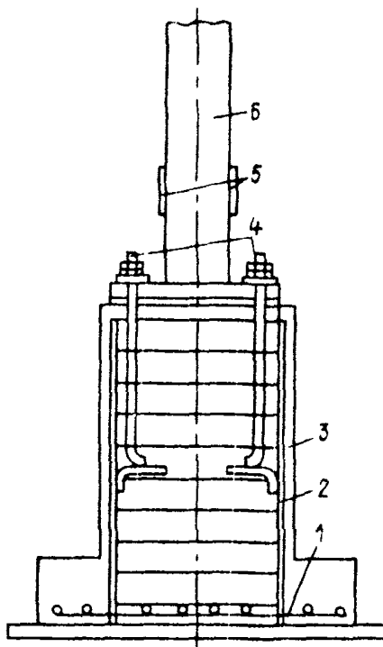
Рис. 2. Соединение металлической колонны с арматурой железобетонного фундамента: 1 — арматура подшивки; 2 — арматура фундамента; 3 — фундамент; 4 — фундаментные болты (не менее двух), соединенные с арматурой фундамента; 5 — пластины для приварки проводников заземления; 6 — стальная колонна
