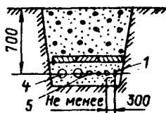
Рис. 5. Прокладка горизонтальных заземлителей в траншее (а) и совместно с кабелем (б): 1 — полоса; 2 — мягкий грунт; 3 — грунт; 4 — силовые кабели; 5 — контрольные кабели
