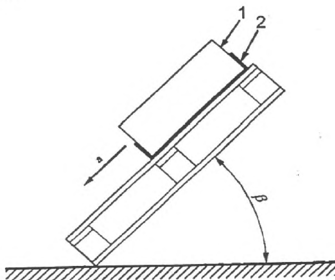
1- коробка размером 400×600 мм; 2- фрикционный материал; β - угол, при котором груз начинает скользить вниз по настилу; а - направление падения
