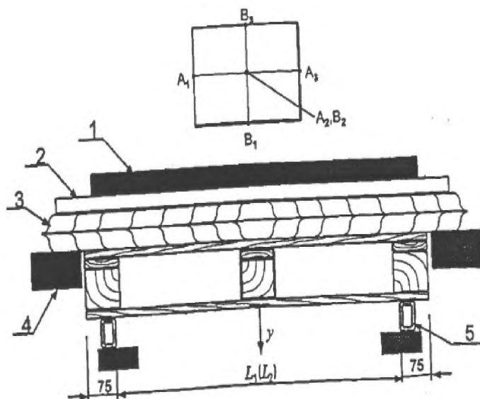
1- статический груз; 2- грузовая платформа; 3 - воздушный амортизатор; 4 - опорная балка воздушного амортизатора; 5 – опоры; y - прогиб
