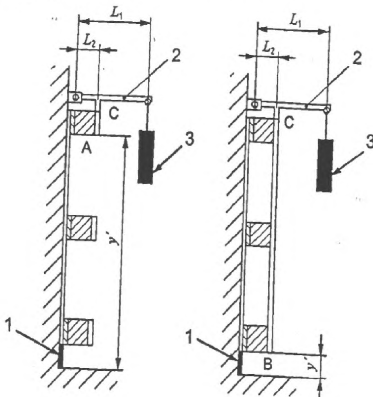
1 – опора; 2- средство нагружения ; 3- груз; у - прогиб; А - С - точки измерения деформации
