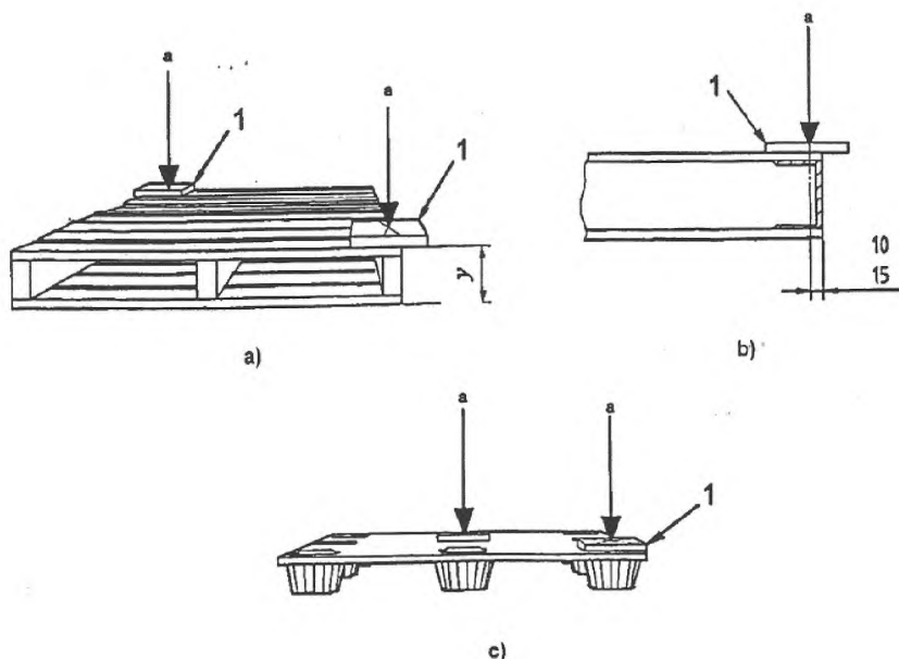
1- средство нагружения; у – прогиб; а - испытательная нагрузка
