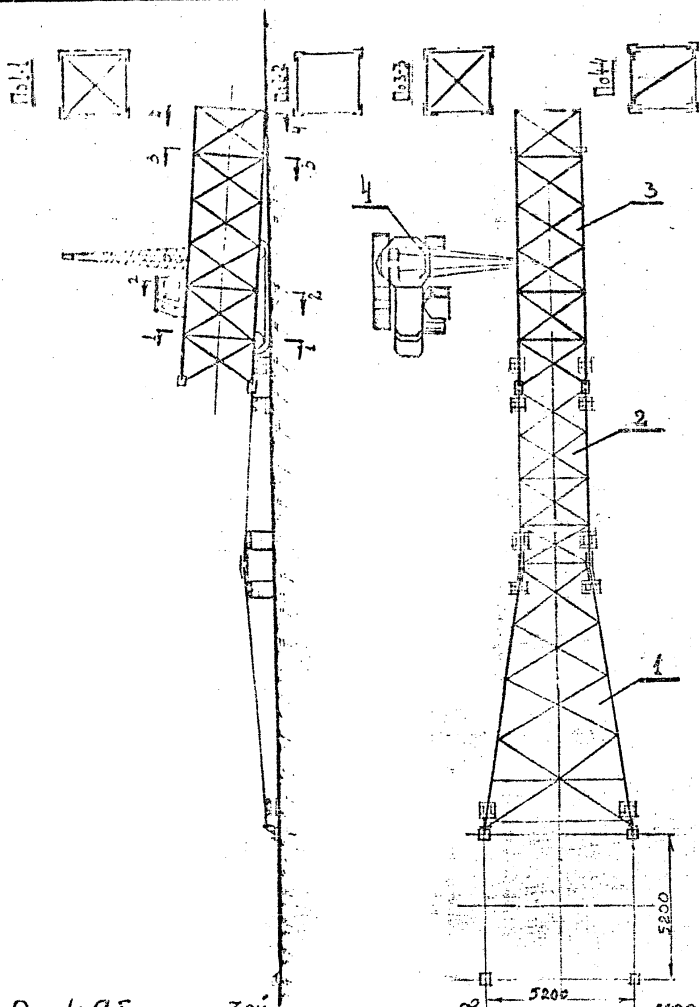
Рис. 43 Сборка 3 ей секции ствола опоры У220-2.
