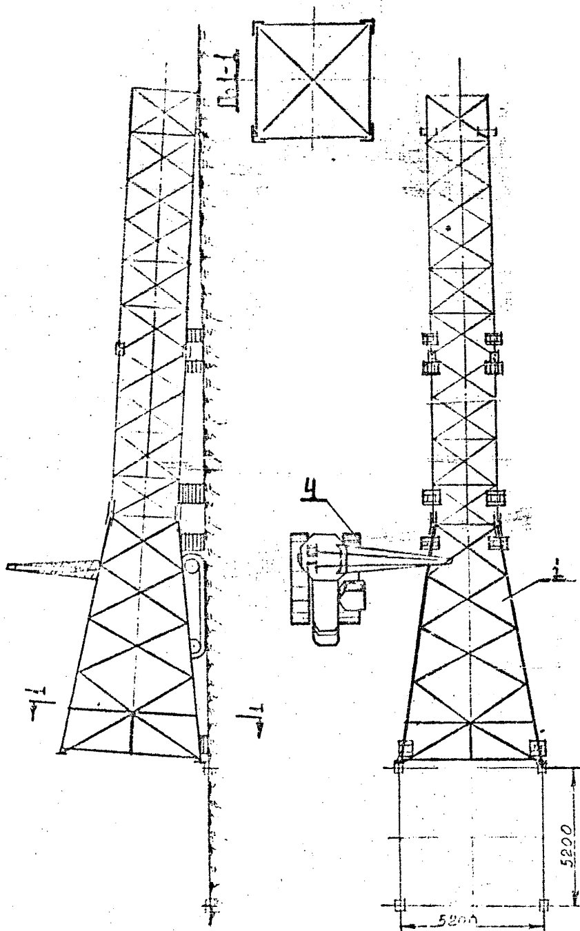
Рис. 15 Сборка 1 ой секции ствкола опоры 4220-2.
