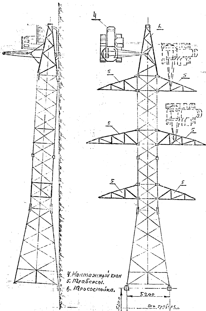
Рис. 46 Пристыковка траверс и трассостойки к стволу опоры 4220-2
