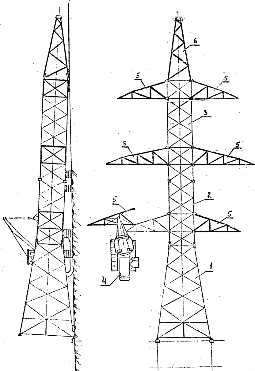
Рис. 8. Пристыковка траверс и тросостойки к стойкам опоры У220-2
