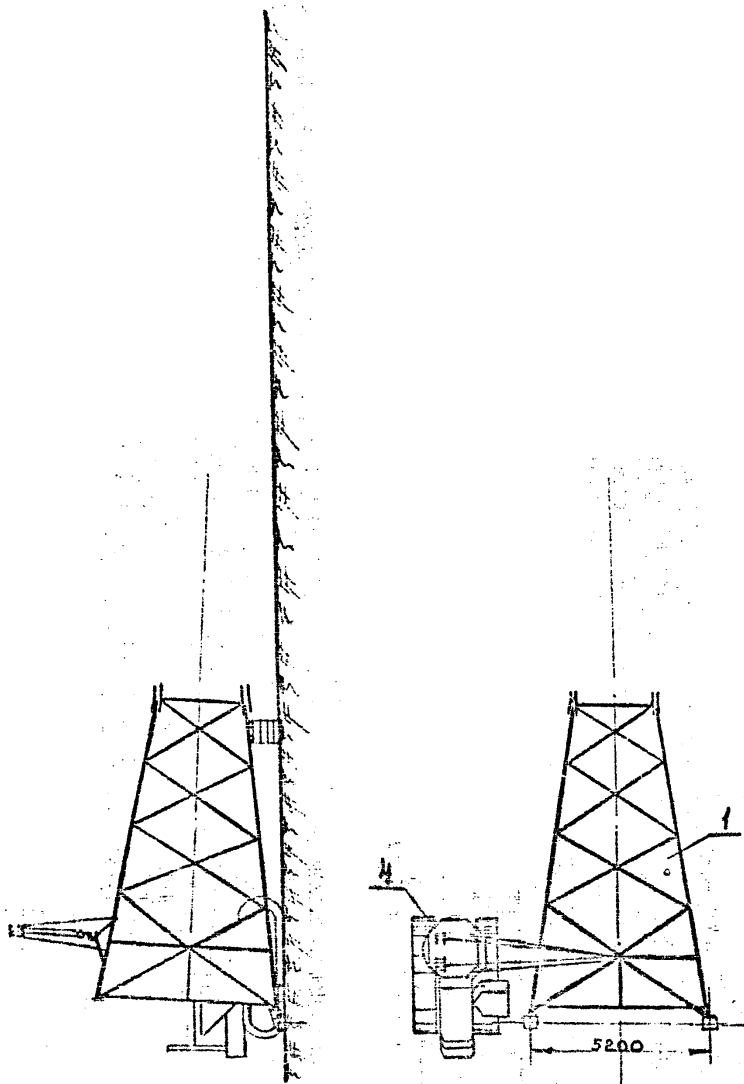
Рис. 49 Сборка 1 ой секции стёла опоры У220-2
