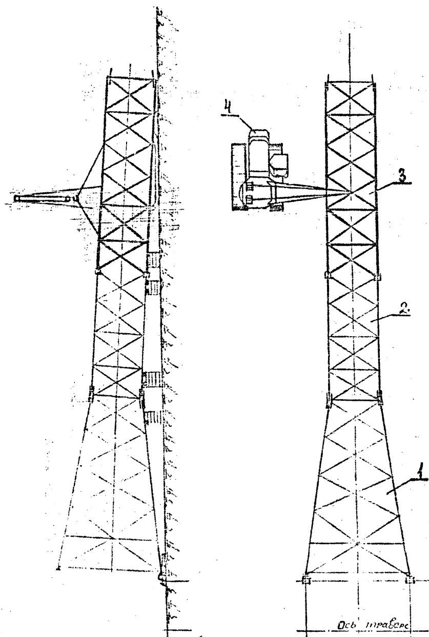
Рис. 51 Пристыковка 3-ей секции ствoла опоры 4220-2 3.3 ая секция опоры Ч. Монтажный кран
