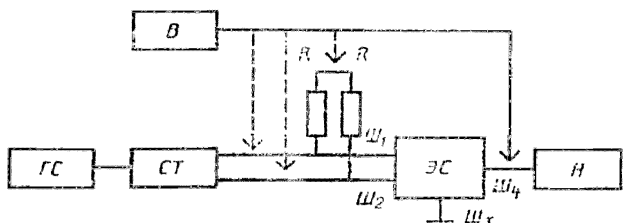
СТ—симметрирующий трансформатор; Ш 1 , Ш 4 —клеммы «Источник радиопомех»; Ш 3 —разъем «Земля»; Ш 4 —разъем «Измеритель радиопомех»
