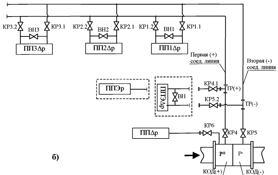
Рис.А. Схемы монтажа РС и подсоединения ППЭ Др и ППЭ Р при проведении контроля ПС Др и ПС Р : а- 1 вариант, б- 2 вариант.
