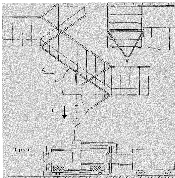
Рис. 6.3. Испытание на прочность марша лестницы
