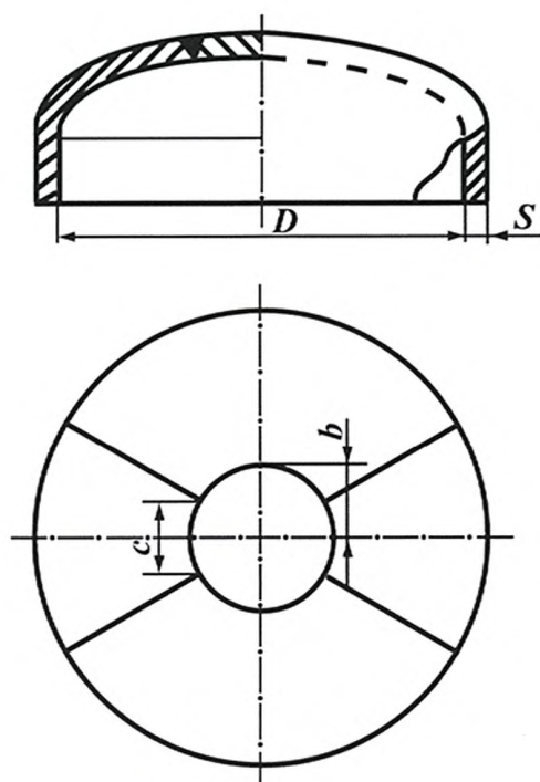
Рис. 8. Расположение радиальных и круговых швов
