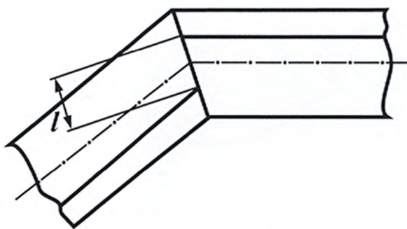
Рис. 6. Расположение сварных соединений в секторных отводах
