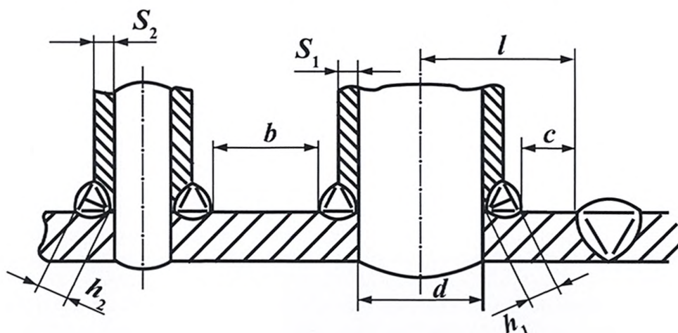
Рис. 9. Расположение сварных соединений приварки патрубков:
