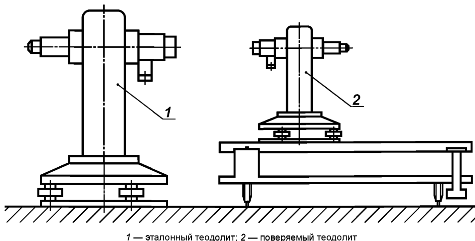
Рисунок 1 — Схема установки эталонного и поверяемого теодолитов
