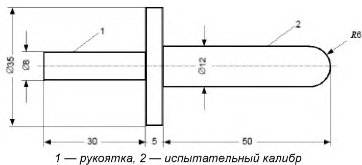
Рисунок 102 – Испытательный щуп
