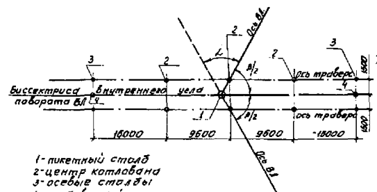
Опоры 4Б330-5-12, 8-6; 4Б330-5-15, 5-6
