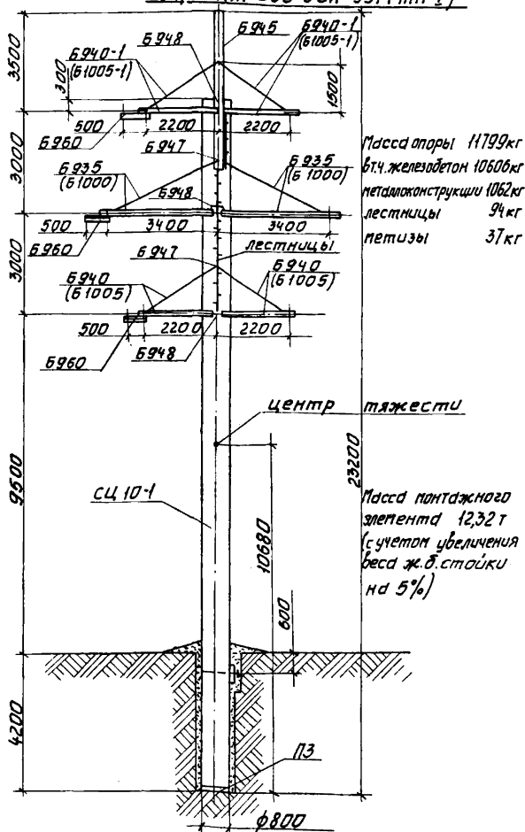
Рис. 0-2 Анкерно-угловая опора 46110-2 (проект СЗД ЭСП 9574 мп-1)
