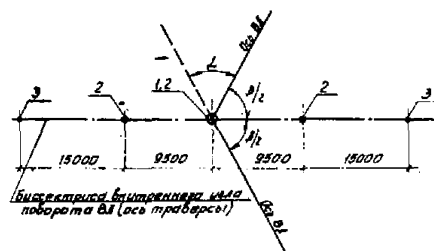
Опоры 4Б330-5-10, 8-3; 4Б330-5-12, 8-3
