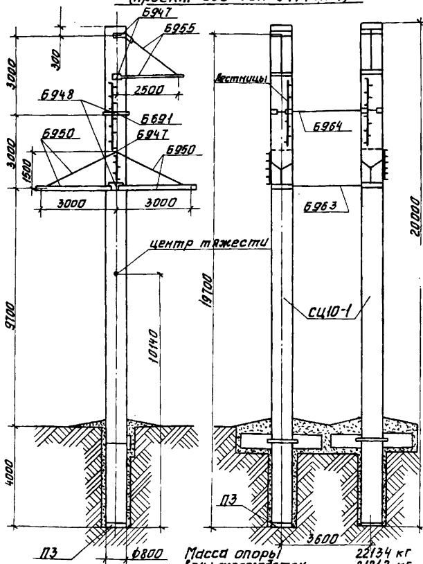
Рис.0-4. Анкерно-угловая опора УБ ИО-9 (проект СЗД ЭСП 9474 тп-1)
