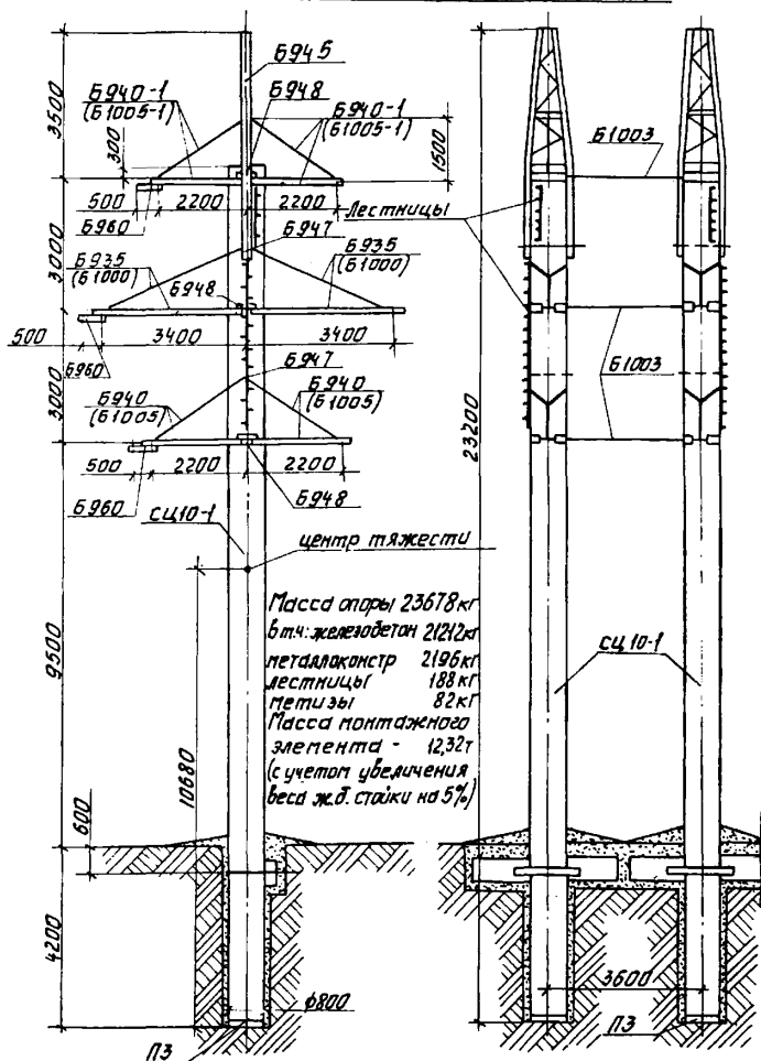
Рис. 0-5. Анкерно-целовая опора ЧБ 110-4 (проект ЭЗП 9574 тм-1)
