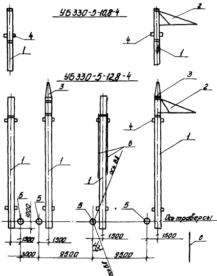
Рис. 5-4. Схемы выкладки и сборки опор 46330-5-128-4 и 46330-5-108-4 при установке крайних КС-5363
