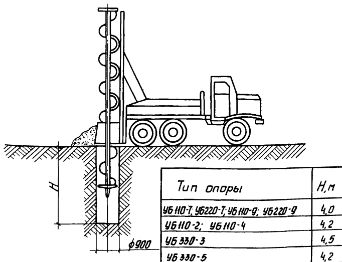
Рис.б-1. Бурение котлованов машиной ПРК-690А с навесным оборудованием УБК-900
