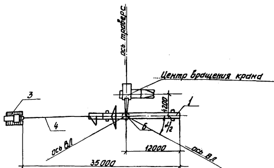
Рис. 7-1. Установка опор 46110-7 и 46220-7 автокраном К-162 и трактором.
