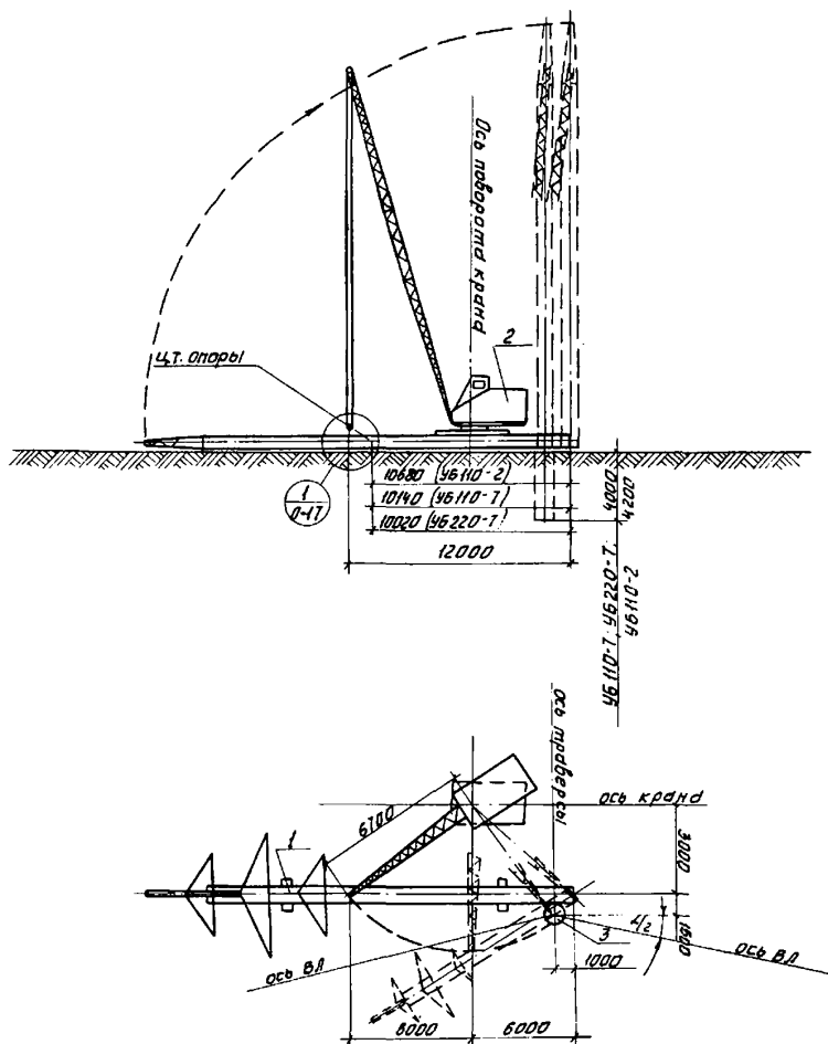
Рис. 8-1. Установка опор УБ110-1, УБ110-2 и УБ220-1 краном КС-5363
