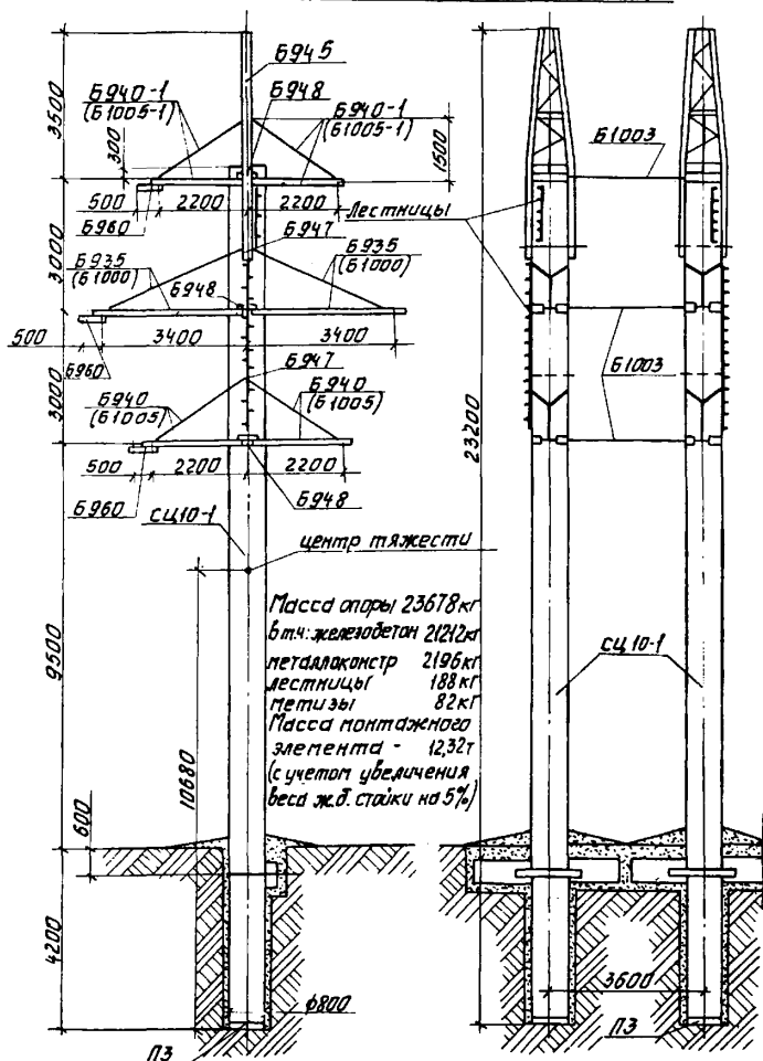
Рис. 0-5. Анкерно-целовая опора ЧБ 110-4 (проект ЭЗП ЭСП 9574 тм-1)
