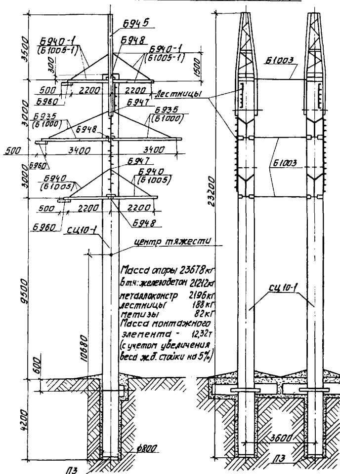
Рис. 0-5. Анкерно-угловая опора ЧБ 110-4 (проект ЭЗП ЭСП 9574 тм-1)
