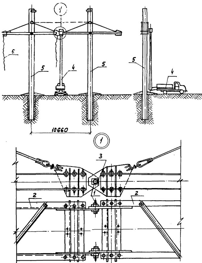
Рис. 13-2. Стыковка тралерс опоры 4Б 330-3
