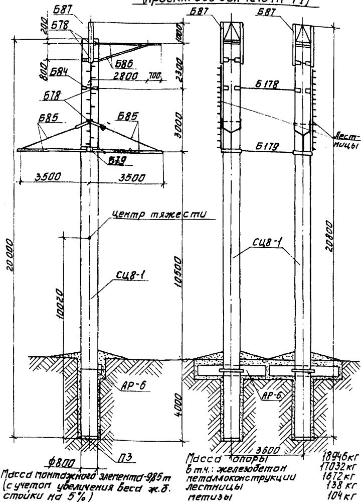
Рис. 0-б. Анкерно-угловая опора 4Б220-9 (проект СЗД ЭСП 7275 тп-т1)
