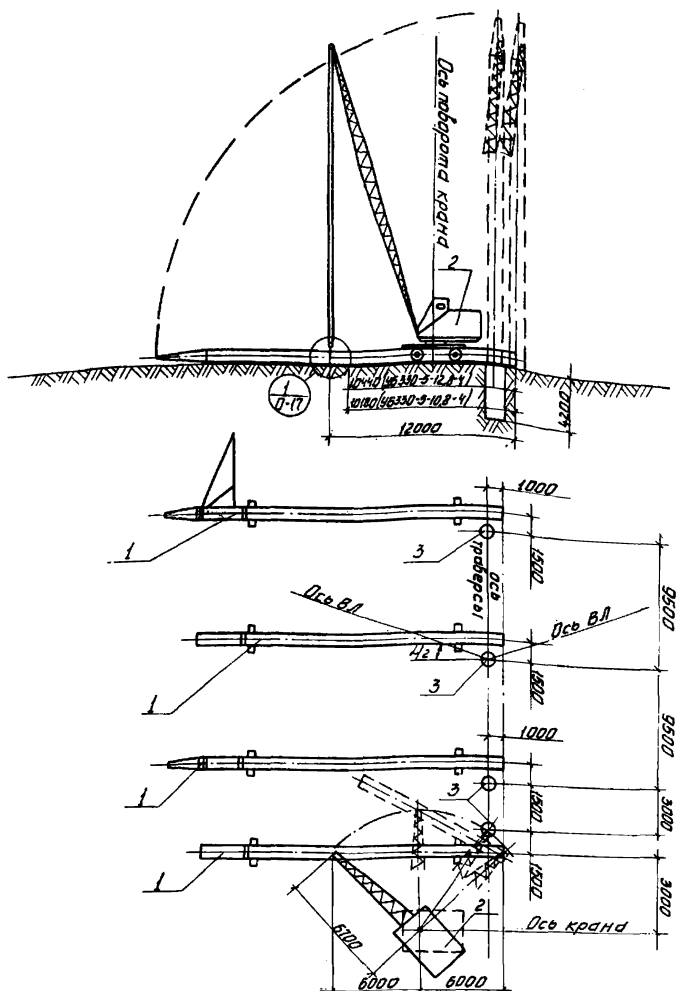
1- Монтажный элемент опоры; 2-Кран КС-5363 Встр.*15м; 3-Котлован L- угол поворота ВЛ
