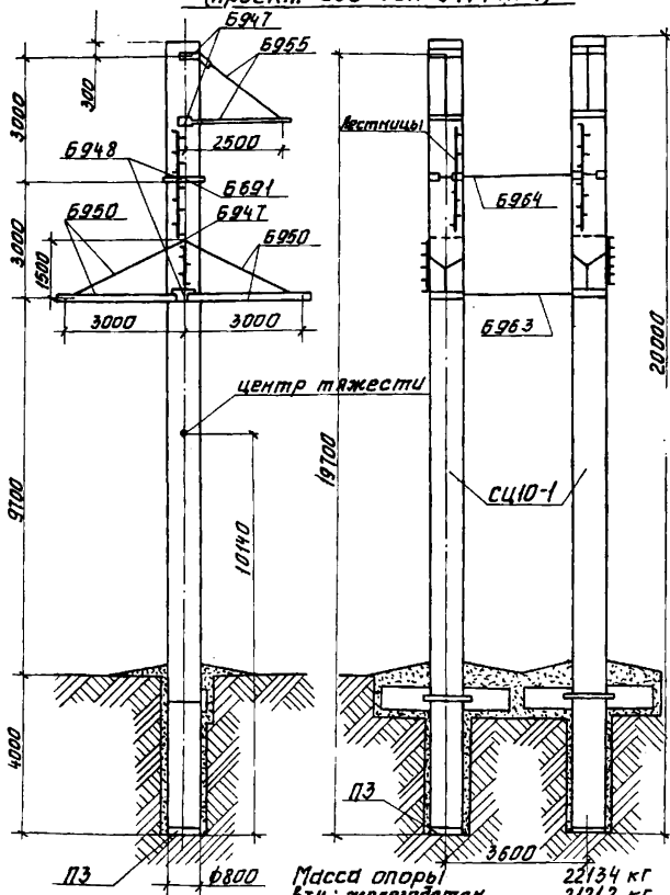
Рис.0-4. Анкерно-угловая опора УБ 110-9 (проект СЗД ЭСП 9474тн-1)
