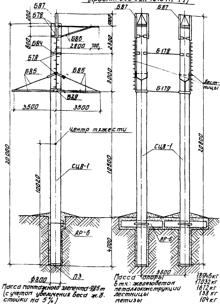
Рис. D-6. Анкерно-угловая опора 4Б220-9 (проект СЗД ЭСП 7275 тп-т1)
